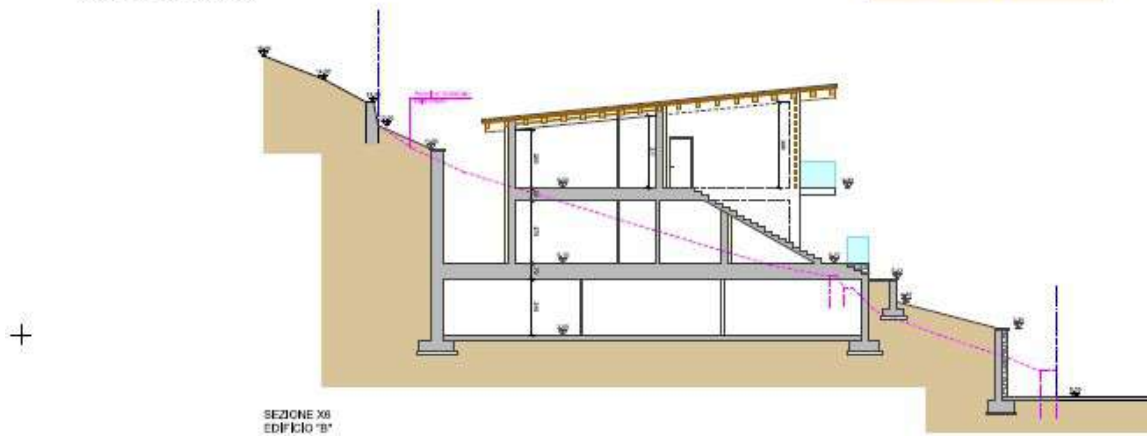
SEZIONE X5 PROSPETTO OVEST EDIFICIO "B"
