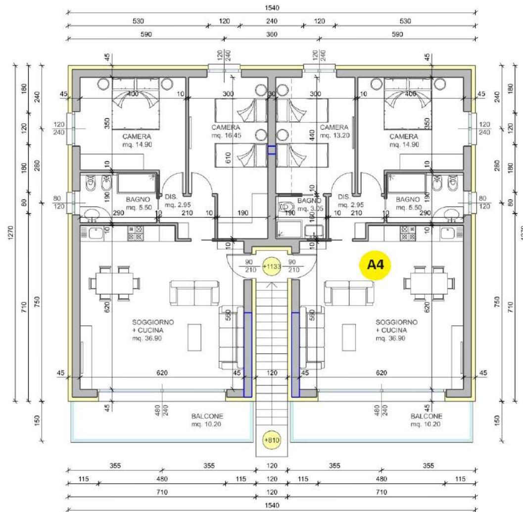
FABBRICATO "A" PIANTA PIANO PRIMO q. +1133
