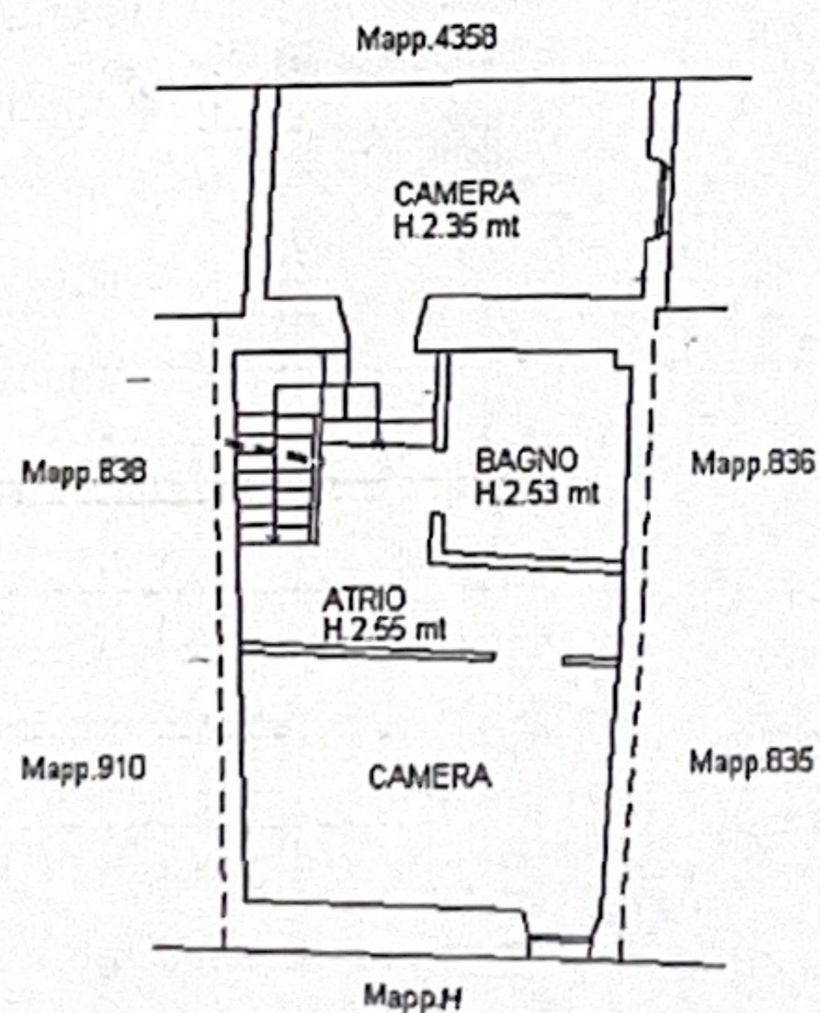
PIANO SECONDO H.2.45 mt
