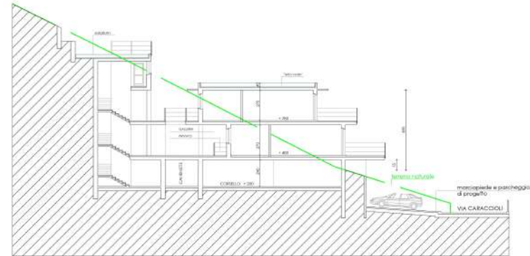
SEZIONE SULLA SCALA 1-100
