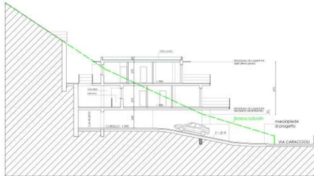
SEZIONE SULLA RAMPA BOX 1-100
