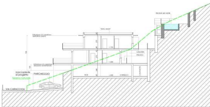
SEZIONE SULLA PISCINA 1:100
