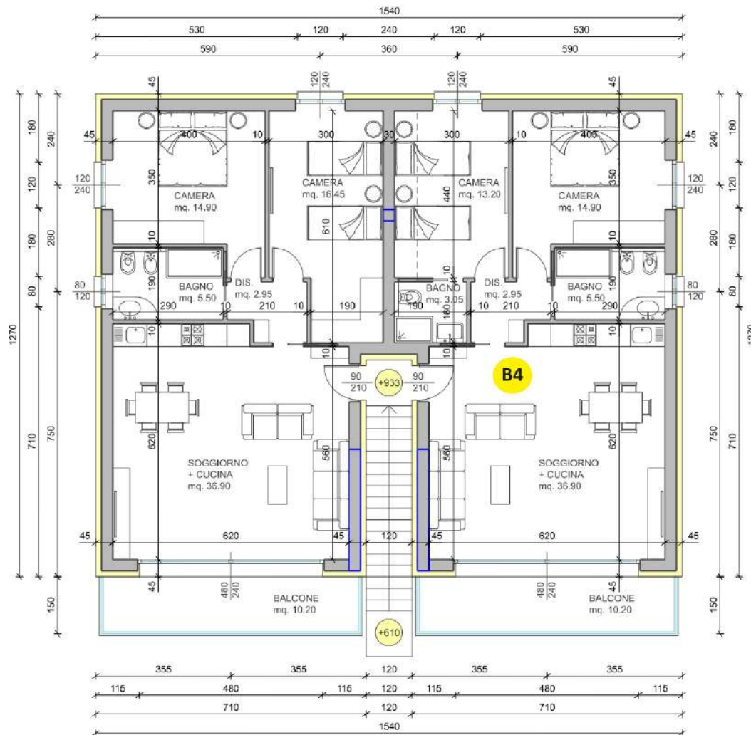
FABBRICATO "B" PIANTA PIANO PRIMO q. +933
